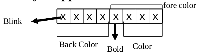
Fig 8 (Attribute Byte)
