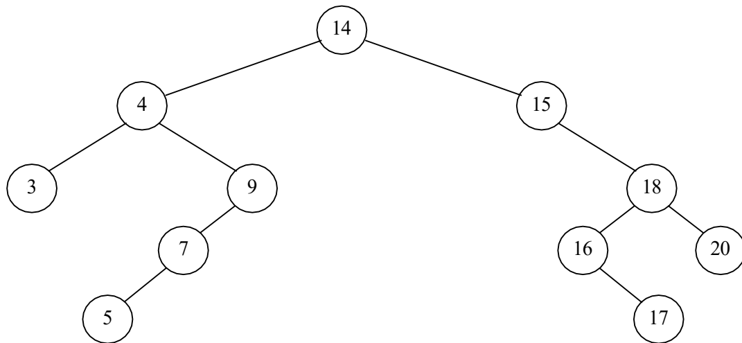
Fig 13.3: Preorder: 14 4 3 9 7 5 15 18 16 17 20
